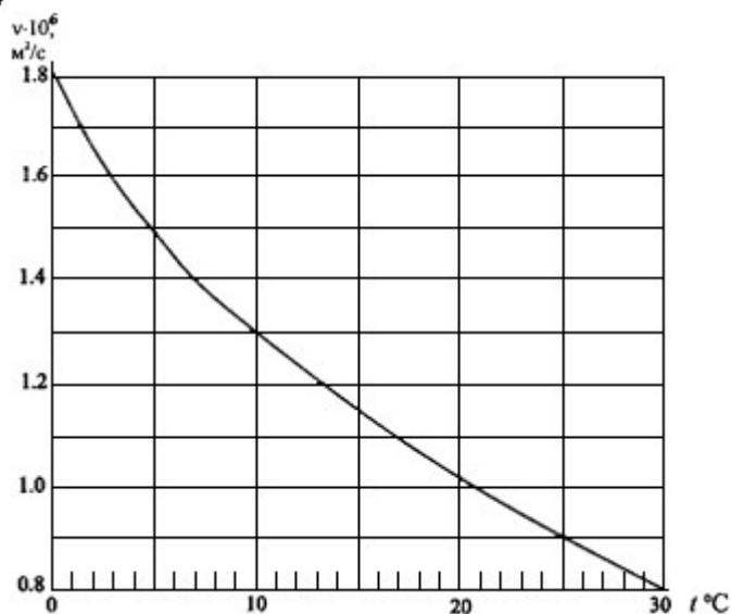
Рис.2. Зависимость кинематического коэффициента вязкости воды \nu от температуры t^\circ\text{C} Режимы обтекания частиц потоком обычно определяют по числу Рейнольдса в несколько иной
