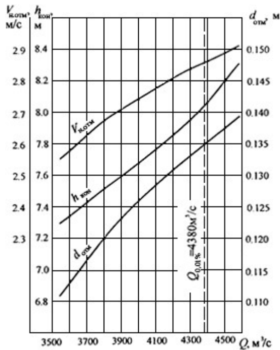
Рис.П3.2. Графики для нахождения параметров самоотмостки русла
