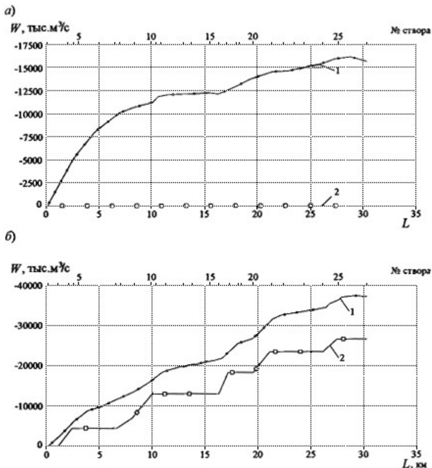
Рис.П4.6. Объемы деформаций (1) и карьерных разработок (2) русла за 1957-1976 гг.:
