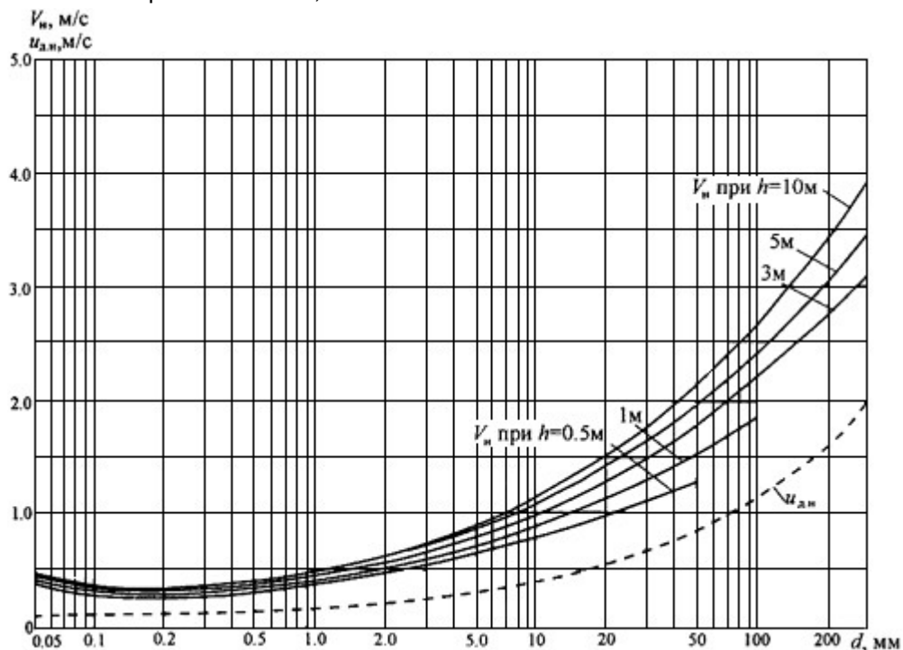
Рис.4. Зависимость неразрывающей скорости V_H несвязных грунтов от диаметра частиц d и глубины потока h (при плотности \rho_s = 2650 кг/м 3 , коэффициенте формы \theta = 0,73 , коэффициенте
