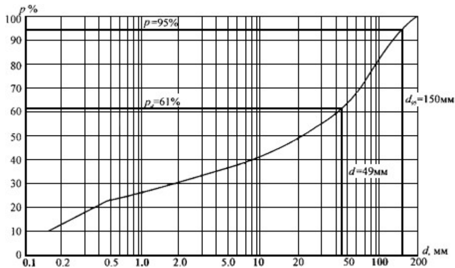
Рис.ПЗ.1. Кривая гранулометрического состава наносов Коэффициент однородности грунта по формуле (86)
