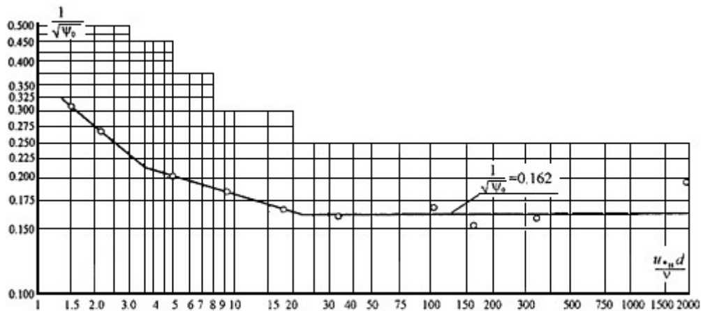
Рис.7. График изменения коэффициента подвижности \frac{1}{\sqrt{\Psi_0}} донных частиц от параметра u_{*н} d / \nu по В.С.Кнорозу
