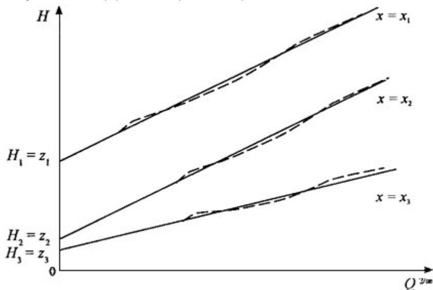
Рис.10. Схема к определению расчетных отметок дна по кривым связи Q = f(H) :
