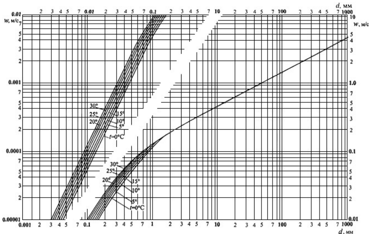
Рис.3. Зависимость гидравлической крупности частиц наносов w от их приведенного диаметра d и температуры воды t °С (при коэффициенте формы \theta = 0,73 )
